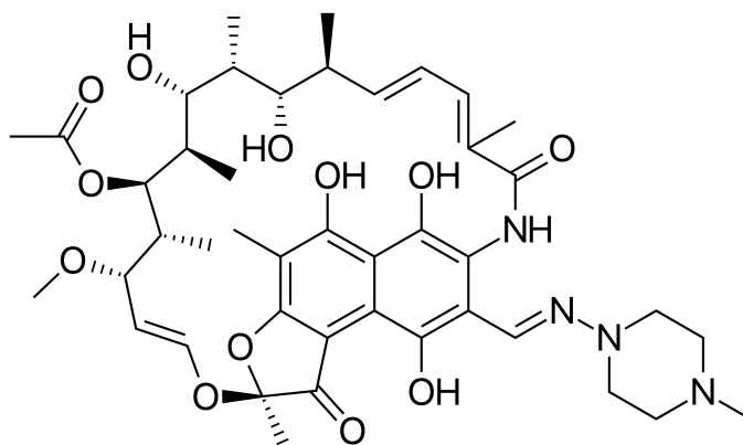
Rifampin
