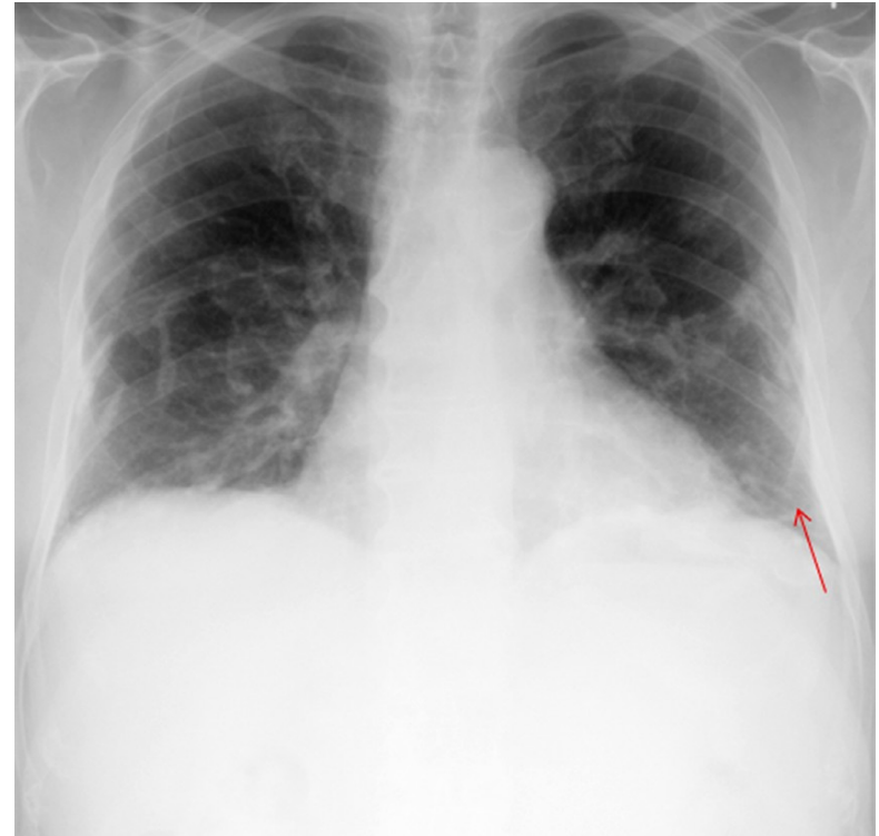
Atelectasis
